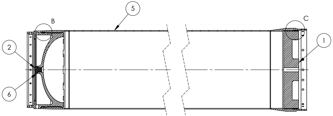
SECCIÓN A-A ESCALA 1 : 5
